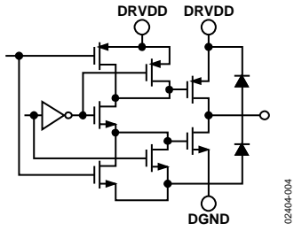
Figure 4. D0-D13, OTR
